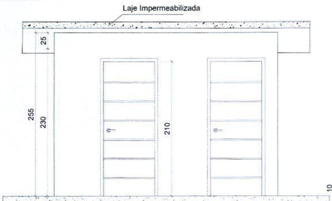
ELEVAÇÃO FRONTAL Sem Escala
