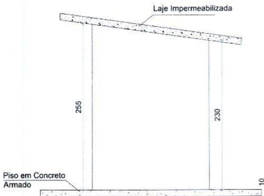
ELEVAÇÃO LATERAL Sem Escala
