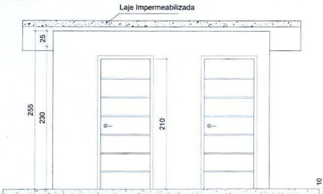
ELEVAÇÃO FRONTAL Sem Escala
